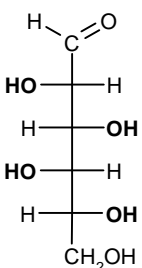
D-idosio
