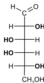
D-galattosio
