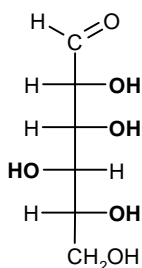
D-gulosio
