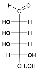
D-talosio
