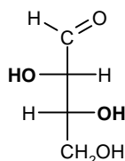
D-treosio
