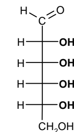
D-allosio
