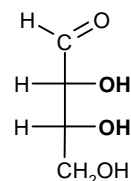
D-eritrosio
