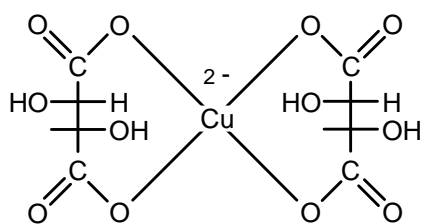
Complesso [Cu(II) (tartrato)] 2- coordinazione planare quadrata
