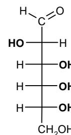
D-altrosio
