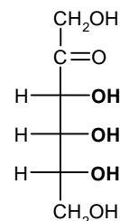
D-psicosio
